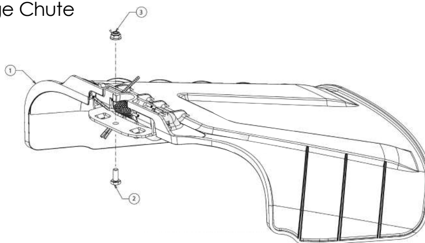
Discharge Chute
