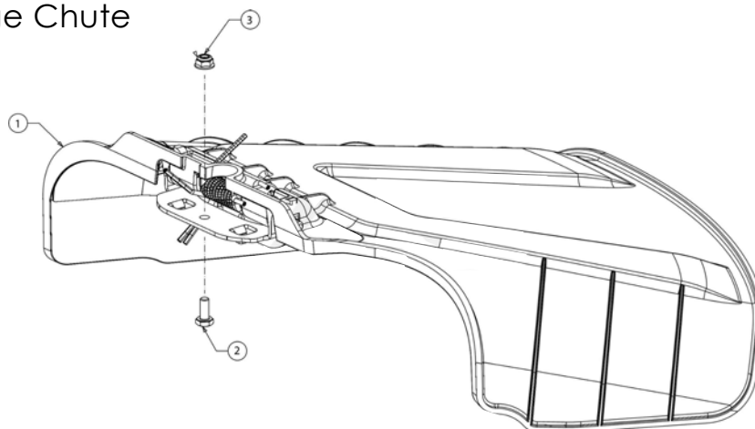
Discharge Chute
