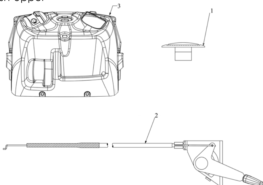
Dash-Upper
